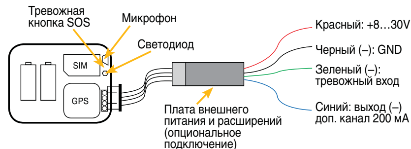
Схема подключения
